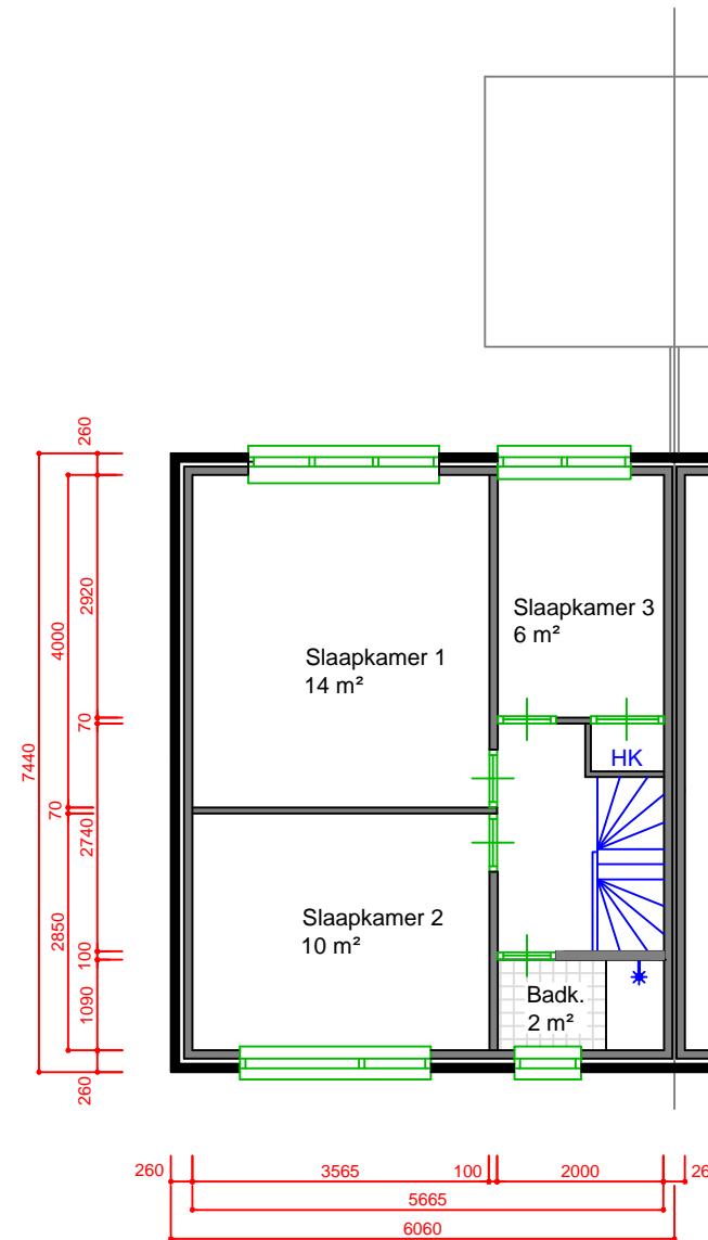
Verdieping
