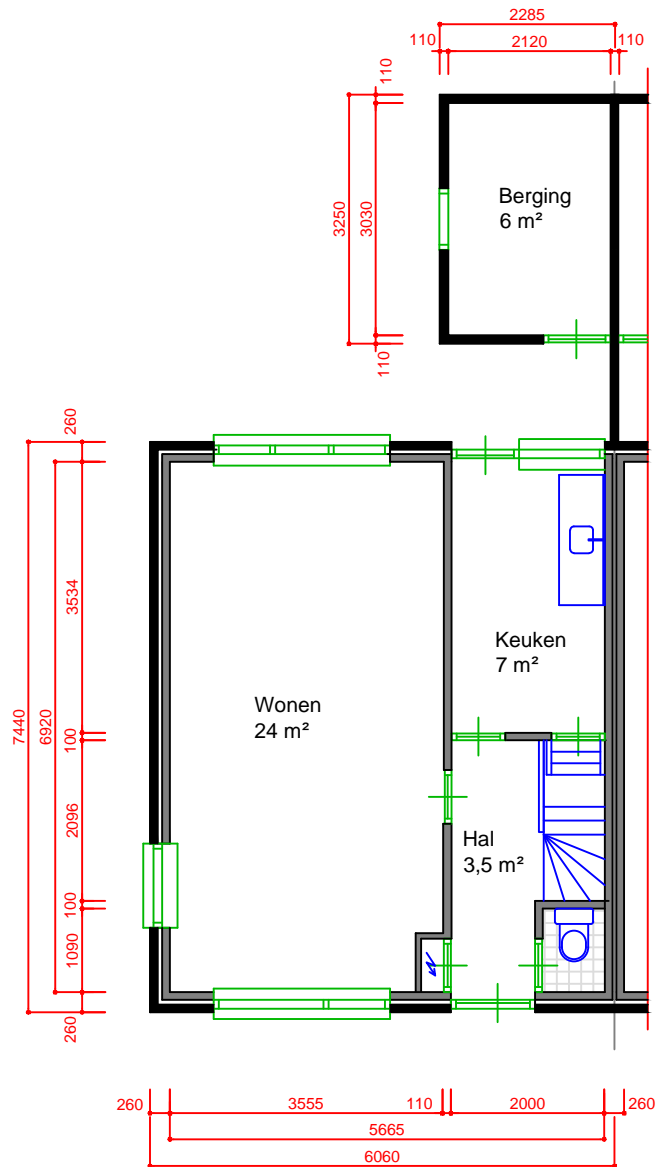
Begane grond
